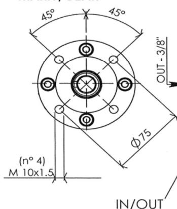
MAR.1/RIDUTTORE MAR.1/GEAR
